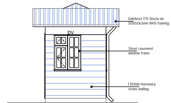
ELEVATION 04
