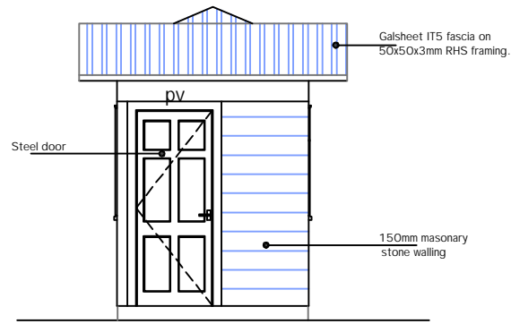
ELEVATION 01
