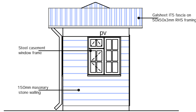
ELEVATION 02
